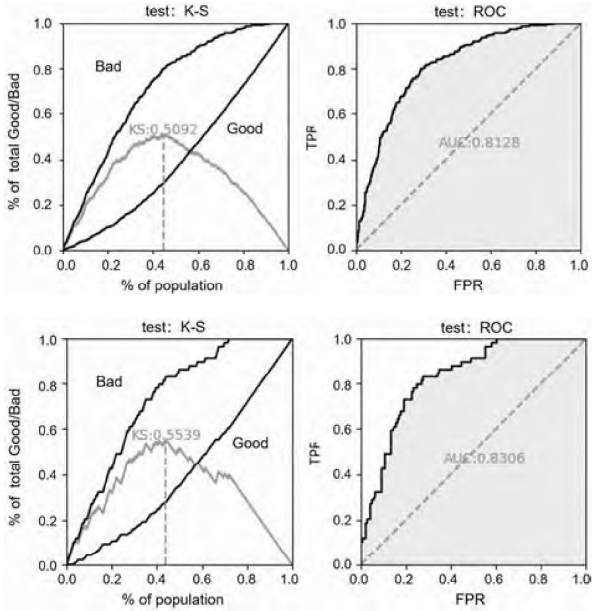
图 6 \alpha=0.98 时特征筛选后模型的 K-S 和 ROC
