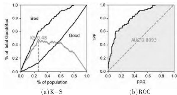
图 1 48 个特征的 LR 模型的 K-S 和 ROC
